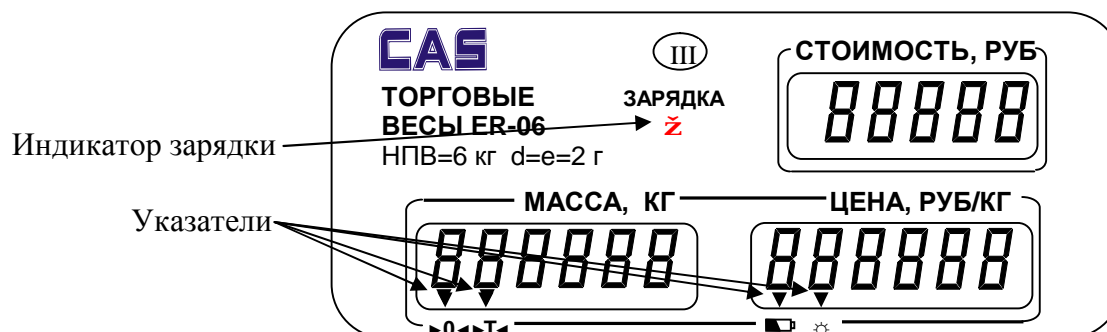
Рисунок 4.2 Вид и назначение элементов панели со стороны покупателя
