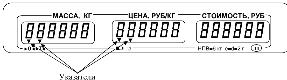
Рисунок 4.2 Вид и назначение элементов панели со стороны покупателя
